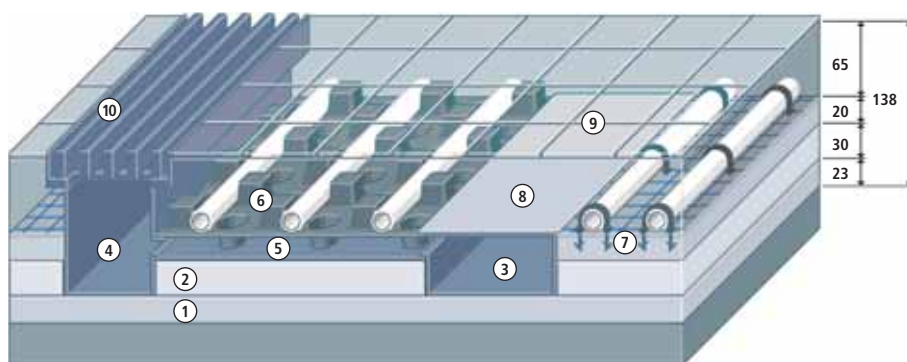
Skladba podlahy proti stejné vytápěnému prostoru
