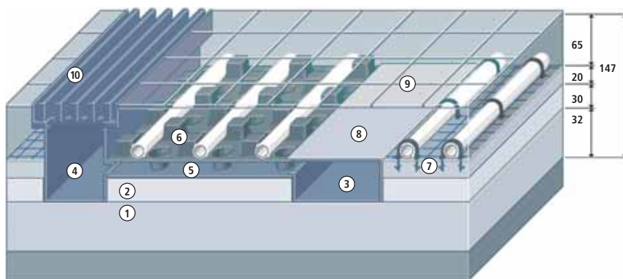
Skladba podlahy proti prostoru s venkovní teplotou
